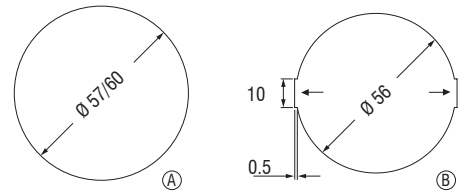
Foro di incasso / Recessed hole / Einbaumaße
